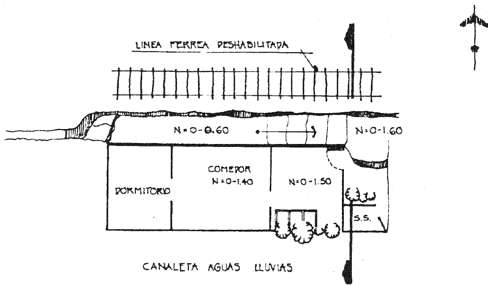
PLANTA ARQUITECTONICA sin escala
